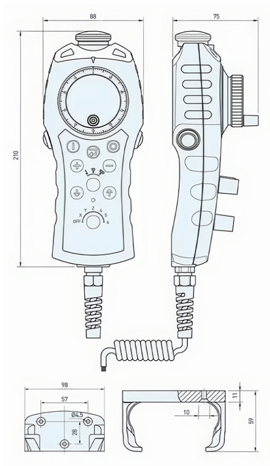
Рисунок 1 — Габаритные размеры пульта.
